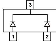
BAT54C Marking : 5C, KL3
